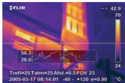
Digital- und Wärmebild eines Verteilerschienensystems in der Produktionshalle
