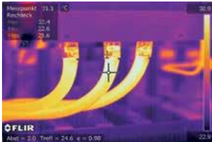
Wärmebild elektrischer Leitungen
