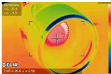
Wärmebild eines Triebwerks; Es braucht schon eine gewisse Erfahrung, um die Wärmebilder eines Flugzeugs richtig "lesen" zu können, da unterschiedliche Materialien verschiedene Emissionsgrade besitzen.
