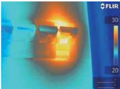
Wärmebild einer überhitzten Sicherung
