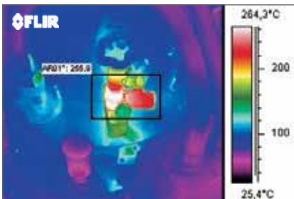
Anzeigearmatur zur Messung des Ölstands des Hauptmotors: nicht isoliert und zu heiß
