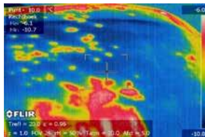
Zahlreiche Schäden oben auf einem Triebwerk, direkt nach der Landung des Flugzeugs aufgenommen
