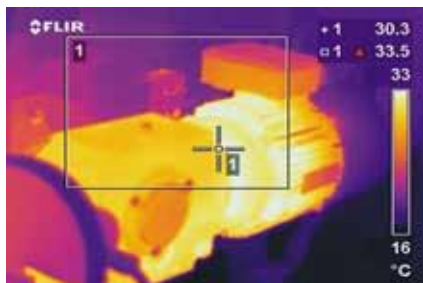
Digital- und Wärmebild eines Motors und eines Getriebes des Gepäck-Handlingsystems in Heathrow
