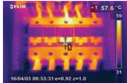
Überhitzte Sicherung
