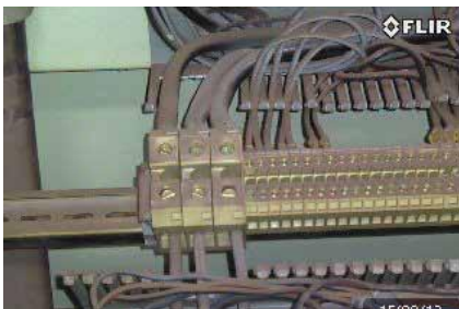
Hier ist eine auffällige Leitung oder Klemme zu sehen. Der Systembetreiber sollte die Ursache abklären.
