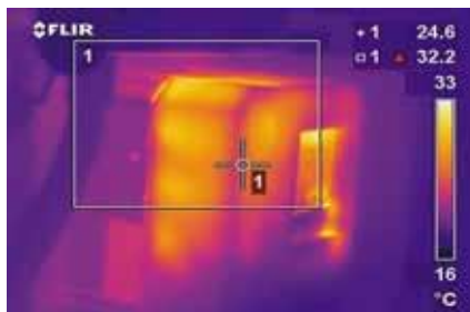
Wärmebild eines Umrichters im Gepäck-Handlingsystem von Heathrow
