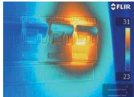
Wärmebild derselben überhitzten Sicherung, jetzt mit der MSX-Funktion. Der Text unter der Sicherung ist lesbar. Dadurch lässt sich die richtige Sicherung problemlos bestimmen und reparieren.
