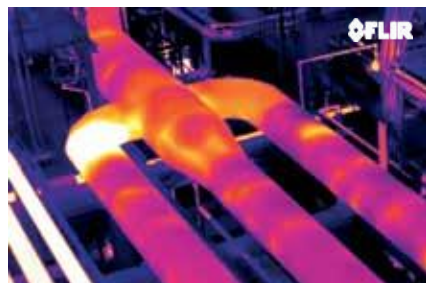
Digital- und Wärmebild einer schadhafte Feuerfestauskleidung in einer Luftleitung
