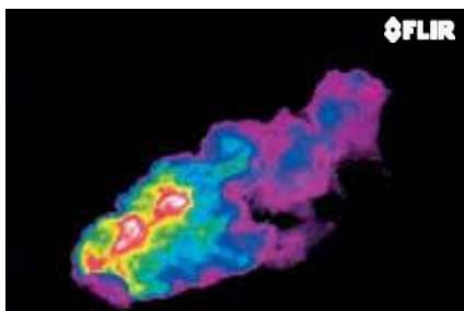
Wärmebild einer Fackel bei Tageslicht
