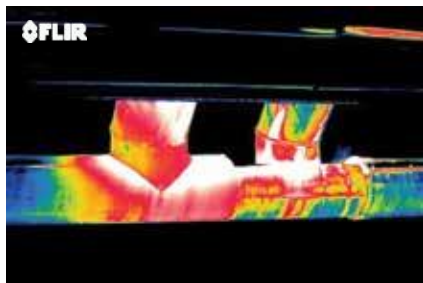
Digital- und Wärmebild einer der Rohrleitungen im Netzwerk. Auf dem Wärmebild ist die fehlerhafte Isolierung eindeutig erkennbar.
