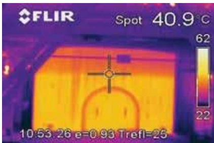
Die Füllstandserkennung von Behältern ist nur eine der Anwendungen der Wärmebildtechnik bei BASF.
