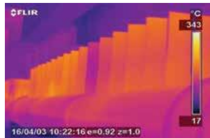
Wärmebildinspektionen der Crack-Leitungen der Anlage zur Produktion von Ammoniaknhydrid.
