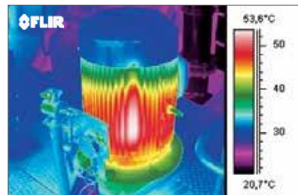
Digital- und Wärmebild einer elektrischen Maschine, die eine Pumpe im Maschinenraum eines Tankers antreibt
