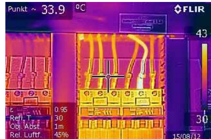
Wärmebild ohne und mit MSX: Im Vergleich zu standardmäßigen Wärmebildern lassen sich mit Hilfe der MSX-Technologie zusätzliche, wichtige Details erkennen.
