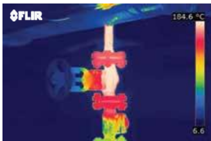
Die Untersuchung enthüllte 150 Problemstellen, die mit der überaus genauen FLIR Wärmebildkamera ausführlich dokumentiert wurden.
