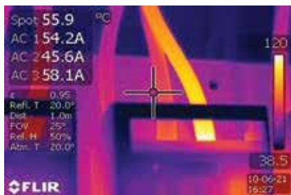
Dank MeterLink werden die mit der Stromzange abgelesenen Werte im Wärmebild angezeigt.
