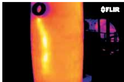
Digital- und Wärmebild eines Defekts einer Feuerfestauskleidung im Innern des Behälters
