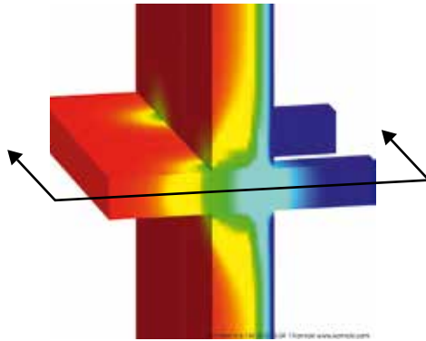
Abbildung 6A: Darstellung einer punktförmigen Wärmebrücke an einem punktförmigen Balkonanschluss. Hier sind von Außen Stahlträger an eine Betondecke angeschlossen. Links ist der warme Innenraum mit roter Oberfläche, rechts der kalte Außenraum mit blauer Oberfläche. An den Innenecken ist durch die gelb-grüne Färbung der Innenoberfläche gut zu erkennen, dass hier an zwei Stellen sehr niedrige Oberflächentemperaturen erreicht werden.
